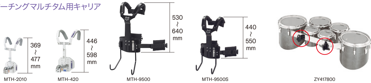
マーチングマルチタム用キャリア
