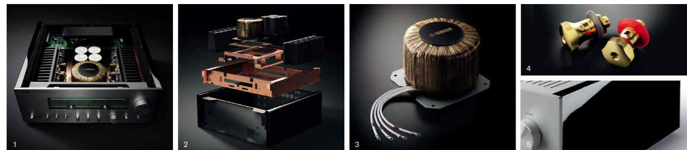
1：リアアンプ部をリアパネル側に配置。パワー部は、中央前方に巨大なトイダル電源トランス、左右に並列MOS-FET採用の出力段を配した完全独立・左右対称レイアウト 2：銅メッキ銅板製の三次元ベースフレームを採用した高剛性・二重構造で振動の影響を全方位的に遮断するリジッド・ストリームライン・コンストラクション 3：二次側巻線を直接取り出して給電ロス排除したカスタムメイドの大型トイダルトランス 4：無垢の真鍮から削り出した大型スピーカー端子 5：ヤマハのグラウンドピアノと同じ塗装・研磨工程で仕上げたピアノブラックのサイドパネル
