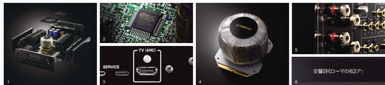
1: メカニカルグラウンド・コンセプトをはじめ、左右対称の筐体設計などHiFiの理想を追求したコンストラクション 2: 音の情報量に加え音楽性を重視し、定評のあるESS社製 高性能32bit D/Aコンバーター「ES9026PRO」 3: ARC(Audio Return Channel) ,CECコントロールに対応し、ジッター対策として専用チューニングを施したHDMI端子 4: トランスの振動を巧みにコントロールする3mm厚の真鍮製ベースプレートを採用したカスタムメイドの大容量トイダル電源トランス 5: 無垢の真鍮から削り出した大型スピーカー端子 6: 入力コンテンツや操作時のボリューム表示などの情報を高品位に表示する日本語対応の有機ELディスプレイ
