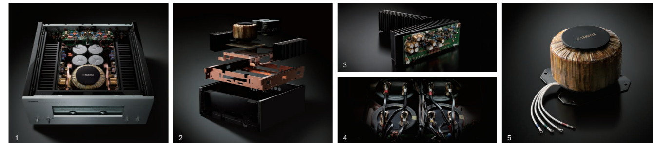
1: 中央前方に巨大なトイダル電源トランス、左右に平行MOS-FET採用の出力段を配置した完全左右対称レイアウト 2: 電源トランスやブロックケミコンなど振動を伴う大型重量部を機構的に接地させるメカニカルグラウンド・コンセプトの導入により進化を遂げた独自のシャーシ構造＝リジッドストリームラインド・コンストラクション 3: 放熱性と制振性を追求した大型ヒートシンクと回路基板を一体化したモノブロック構造 4: 大電流経路の主要配線をすべてネジ止め結線とするなどローインピーダンス設計を徹底 5: 二次側巻線を直接取り出して給電ロスを排除したカスタムメイド容量1200VAの大型トイダル電源トランス
