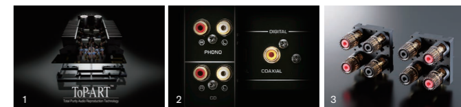
1：「ToP-ART」(Total Purity Audio Reproduction Technology)に基づき設計された左右対応の基板レイアウト&筐体設計 2：金メッキ加工を施し、音質の劣化を低減する入力端子群 3：バナナプラグ対応、金メッキ大型スピーカーターミナル
