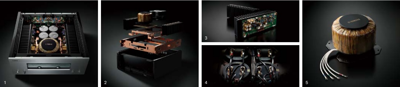
1：中央前方に巨大なトロイダル電源トランス、左右にパラレルMOS-FET採用の出力段を配置した完全左右対称レイアウト 2：電源トランスやブロックケミコンなど振動を伴う大型重量パーツを機構的に接地させるメカニカルグラウンド・コンセプトの導入により進化を遂げた独創的シャーシ構造＝リジッドストリームラインド・コンストラクション 3：放熱性と制振性を追求した大型ヒートシンクと回路基板を一体化したモノブロック構造 4：大電流経路の主要配線をすべてネジ止め結線とするなどローインピーダンス設計を徹底 5：二次側巻線を直接取り出して給電口を排除したカスタムメイド 容量1200VAの大型トロイダル電源トランス
