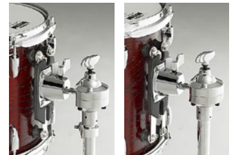
CT-9006~ CT-9010用マウント (ゴムスペーサー3点支持) CT-9012~ CT-9016用マウント (ゴムスペーサー4点支持)
