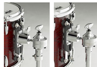
CT-9006～CT-9010用マウント (ゴムスペーサー3点支持) CT-9012～CT-9016用マウント (ゴムスペーサー4点支持)
