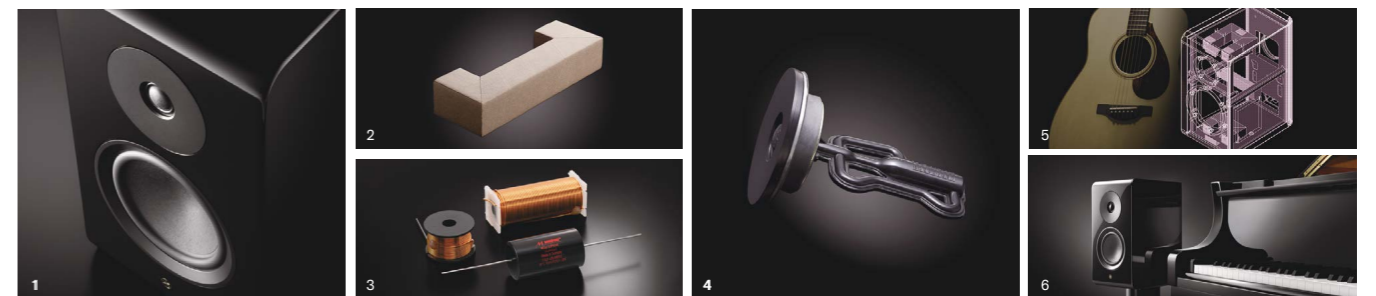
1: 3cmツイーター / 16cmウーファー(NS-600Aは、13cm)、それぞれの特性に合わせて素材の配合を最適化した専用設計のハーモニアスダイアフラム 2: 音響特性に合わせて専用設計されたアコースティックアブソーバー 3: ドイツ ムンドルフ社製オーディオコンデンサー「MCap SUPREME Classic」など、厳選した高級パーツを使用したネットワーク回路 4: 中央のメインチャンバーで発生した共振を長さが異なる左右2本の共鳴管で打ち消すR.S.チャンバー 5: 楽器の研究・開発などに用いられるレーザー振動計と高度なFEM(Finite Element Method)解析を導入した最適な補強&キャビネット構造 6: ヤマハのグランドピアノと同じ専用塗料と下地材、研磨工程によって仕上げた黒鏡面ピアノフィニッシュ
