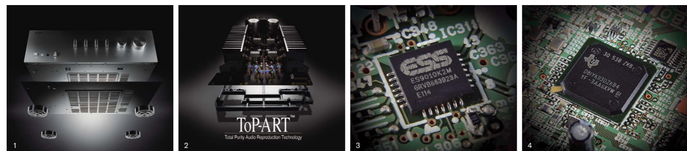
1: 制振・高剛性設計のシャーシに、1mm厚の鉄製プレートを組み合わせたダブルボトムコンストラクション 2: 音楽信号の流れに忠実であることを追求した“ToP-ART”(Total Purity Audio Reproduction Technology)に基づき設計された左右対応の基板レイアウト&筐体設計 3: DSD 11.2MHz、PCM 384kHz/32bit再生に対応した32bit・2ch仕様の高性能D/Aコンバーター「SABRE 32」(ES9010K2M) 4: IC内部にマスタークロックを持ち、PC側のマスタークロックとは同期せず高精度に信号を伝送できるヤマハオリジナルのUSBデバイスコントローラー
