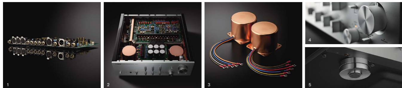
1: Lチャンネル用基板(上側)とRチャンネル用基板(下側)を鏡に映したような対称形に配置。プリントパターン面を向かい合わせてチャンネル間のグラウンドの距離を限りなくゼロに近づけるブックマッチ・コンストラクション 2: 本体前側の左右端に2基の電源トランスを据え、その間に6個のブロックメコンを搭載したメインレギュレーター基板。最短距離かつ左右等長に給電されるようにその背後に配置されたメイン基板 3: 巻線からダイレクトに給電ワイヤーを引き出し、低インピーダンス化に貢献する真鍮ラグを採用した銅メッキケース封入のトイダル電源トランス 4: アルミ削り出しの真鍮高レバースイッチ。軸受部にボールベアリングを採用したボリュームノブ 5: スパイクを内蔵することで通常設置でもピンポイント支持効果を得ることができるC-5000/M-5000専用設計のレグ
