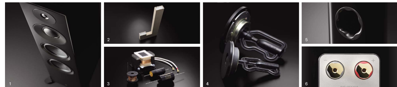
1: 3cmツイーター / 8cmミッドレンジ / 16cmウーファー、各ユニットの特性に合わせて素材の配合を最適化したハーモニアスダイアフラムを採用した3ウェイ4スピーカー構成 2: NS-2000Aの音響特性に合わせて専用設計されたアコースティックアブソーバー 3: ドイツ ムンドルフ社製オーディオコンデンサー「MCap SUPREME Classic」など、厳選した高級パーツを使用したネットワーク回路。内部配線の全てに新世代の銅導体=PC-Triple C(ピーシートリアルシー)を使用 4: 中央のメインチャンバーで発生した共振を長さが異なる左右2本の共鳴管で打ち消すR.S.チャンバー 5: ポートノイズを低減し、S/N感を向上させる独自のツイステッドフレアポート 6: 自然な聴き心地にこだわりシングルワイヤリングを採用した真鍮削り出しのスピーカーターミナル
