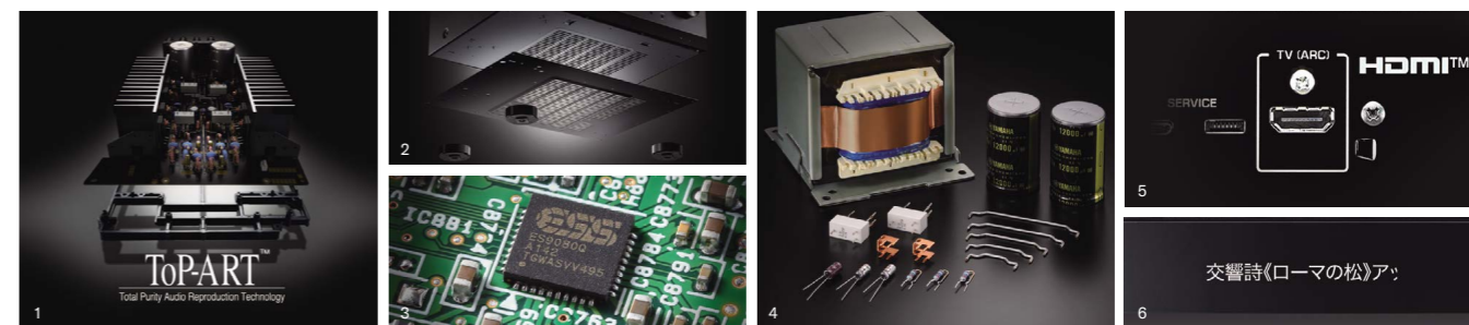
1: 独自の特殊樹脂フレーム“アートベース”を搭載し、“ToP-ART”に基づき設計された左右対称の筐体 2: 底面に1mm厚の鉄板を加え、制振・耐振性能をさらに強化したダブルボトムシャーシ 3: 高調波歪特性に優れ、定評のあるESS社製 32bit D/Aコンバーター「ES9080Q」 4: カスタムメイドの大型E1トランスや大容量ブロックケミコン(12,000μF×2本)、アムトランス社製の抵抗など厳選した高音質パーツ 5: ARC(Audio Return Channel)・CECコントロールに対応しジッター対策として専用チューニングを施したHDMI端子 6: 入力コンテンツや操作時のボリューム表示などの情報を高品位に表示する日本語対応の有機ELディスプレイ
