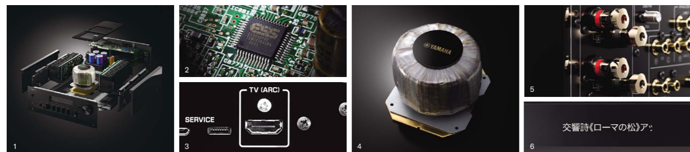
1: メカニカルグラウンド・コンセプトをはじめ、左右対称の筐体設計などHiFiの理想を追求したコンストラクション 2: 音の情報量に加え音楽性を重視し、定評のあるESS社製 高性能32bit D/Aコンバーター「ES9026PRO」 3: ARC(Audio Return Channel)・CECコントロールに対応し、ジッター対策として専用チューニングを施したHDMI端子 4: トランスの振動を巧みにコントロールする3mm厚の真鍮製ベースプレートを採用したカスタムメイドの大容量トイダル電源トランス 5: 無垢の真鍮から削り出した大型スピーカー端子 6: 入力コンテンツや操作時のボリューム表示などの情報を高品位に表示する日本語対応の有機ELディスプレイ
