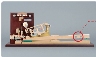
グランドピアノの鍵盤機構
