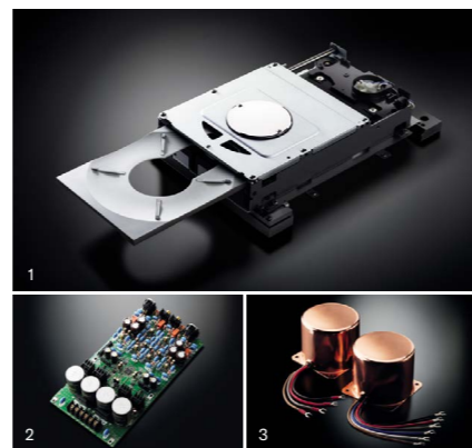
1：水平の微調整を行い取り付けられるCDドライブメカニズム 2：アナログ系電源回路をオーディオ基板上に展開して給電ロスを排除 3：防磁・制振効果の高い銅メッキケースに封入した専用設計のトロイダル電源トランス
