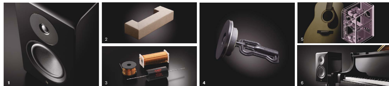
1: 3cmツイーター / 16cmウーファー(NS-600Aは、13cm)、それぞれの特性に合わせて素材の配合を最適化した専用設計のハーモニアスダイアフラム 2: 音響特性に合わせて専用設計されたアコースティックアブソーバー 3: ドイツ ムンドルフ社製オーディオコンデンサー「MCap SUPREME Classic」など、厳選した高級パーツを使用したネットワーク回路 4: 中央のメインチャンバーで発生した共振を長さが異なる左右2本の共鳴管で打ち消すR.S.チャンバー 5: 楽器の研究・開発などに用いられるレーザー振動計と高度なFEM(Finite Element Method)解析を導入した最適な補強機&キャビネット構造 6: ヤマハのグランドピアノと同じ専用塗料と下地材、研磨工程によって仕上げた黒鏡面ピアノフィニッシュ
