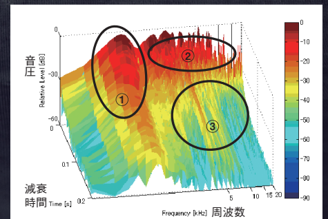
A.R.E.を適用したバイオリン (YVN500S)
