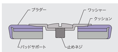
ストロビンガーフェニックス™パッド (YFL-700/600シリーズ)
