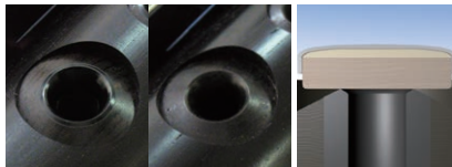
800Lシリーズのトーンホール | 従来モデルのトーンホール
