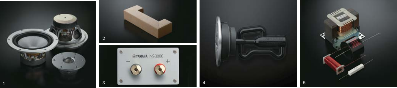
1：ダイヤフラムとサラウンドとを継ぎ目なく一体成型した100% ZYLON®16cm口径コーン型ウーファーと(左・上)と100% ZYLON®3cm口径ソフトドーム型ツイーター(右) 2：NS-3000の音響特性に合わせて専用設計された新形状の「アコースティックアブソーバー」 3：自然な聴き心地にこだわリシングルワイヤリングとした真鍮削り出しの高品位スピーカーターミナル 4：中央のメインチャンバーで発生した共鳴を長さが異なる左右2本の共鳴管で打ち消すR.S.チャンバー 5：ドイツ ムンドルフ社製のオーディオコンデンサー「MCap SUPREME EVO」や高音質アッテネーター「MResist SUPREME」Jなど、厳選した最高級パーツを使用したネットワーク回路
