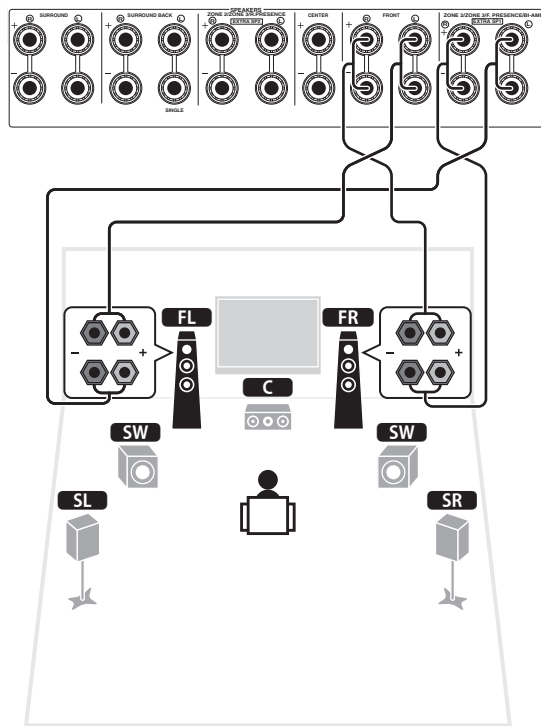
本機（背面）
