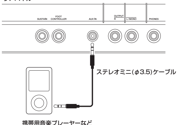
リアパネル
