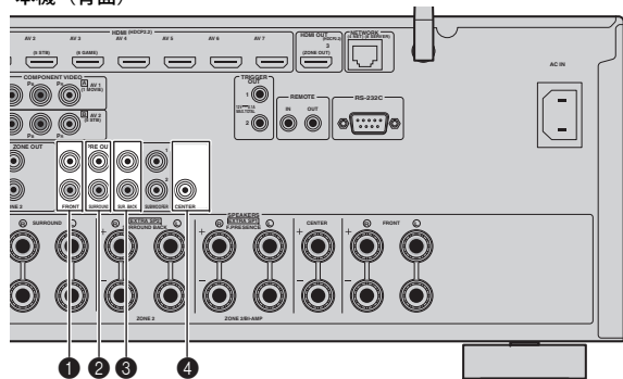
本機（背面）
