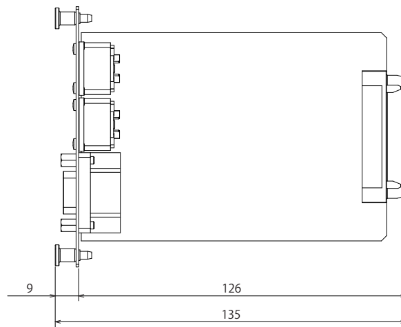
上面図
