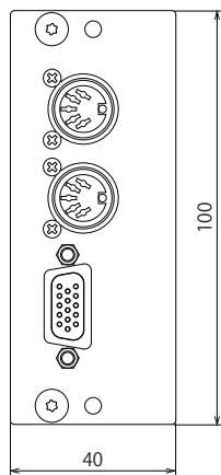
正面図
