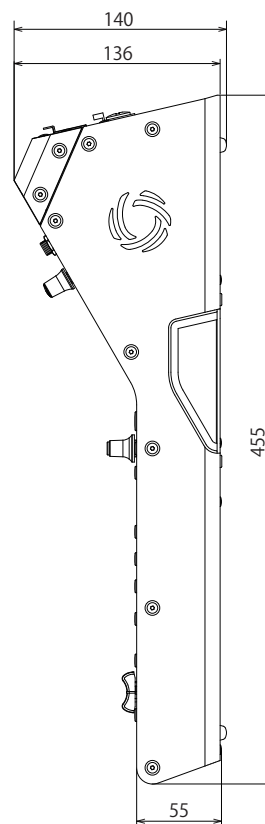
側面図
