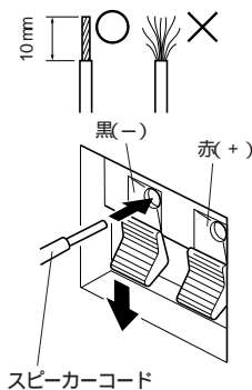
<アンプのスピーカー端子>
