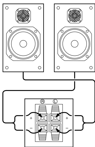
<アンプのスピーカー端子>
