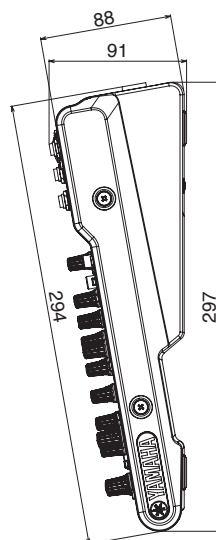
側面図
