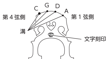
【テールピース側から見た駒】
