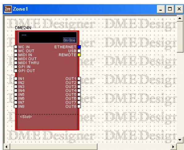
スロットにI/Oカードが接続されていないDME24N
