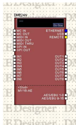
スロットにI/Oカードが接続されているDME24N
