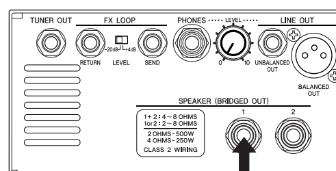
Toma de salida de altavoz del amplificador
