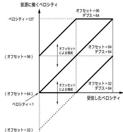
オフセットによるペロシティカーブの変化 (デプス=64で一定にしたとき)
