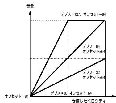
デプスによるペロシティカーブの変化 (オフセット=64で一定にしたとき)
