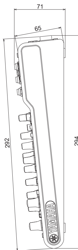
側面図
