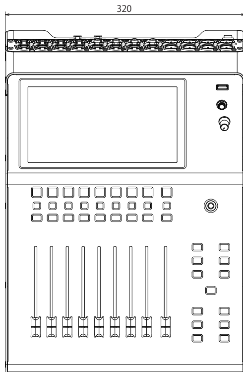
上面図
