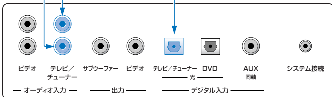
YSP-800(背面)
