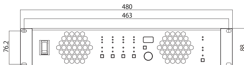
正面図
