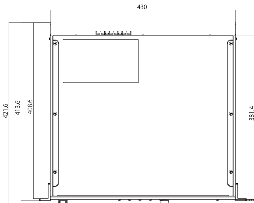
上面図
