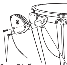
チューニングインジケータ固定ボルト
