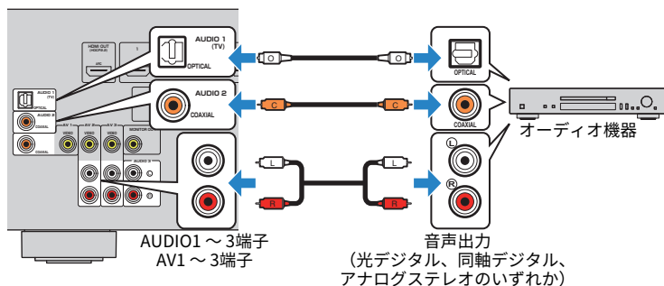
本機（背面）
