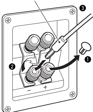
バナナプラグ
