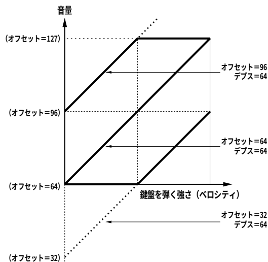
デプスによるベロシティカーブの変化 (デプス=64で一定にしたとき)
