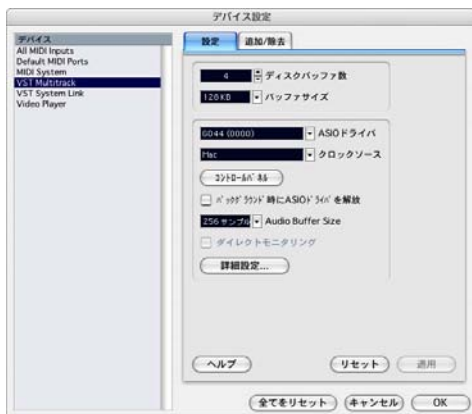
Cubase LE
