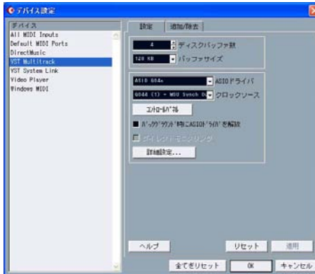
Cubase LE
