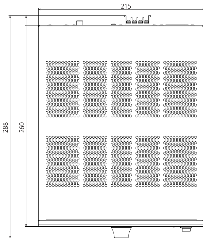
上面図
