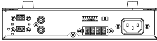
背面図
