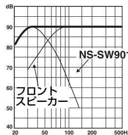
周波数特性イメージ*
