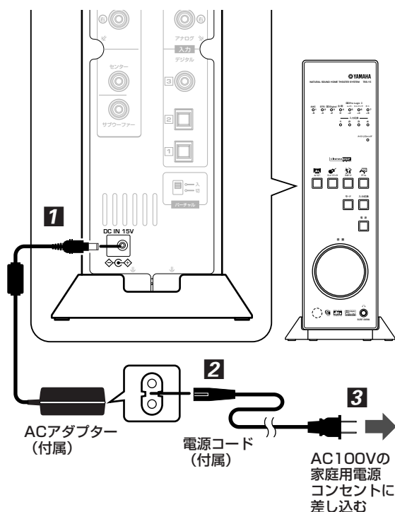
アンプユニット背面
