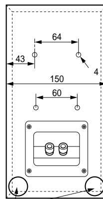
防振用スピーカー貼付位置
