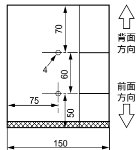
<スピーカー底面ネジ位置>
