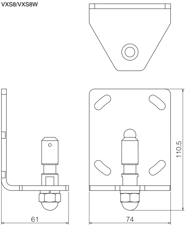
VXS8/VXS8W
