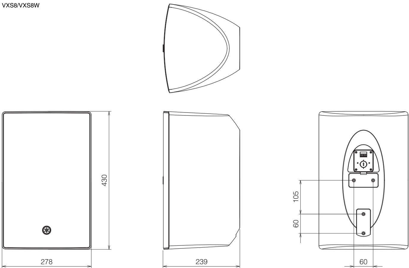
VXS8/VXS8W
