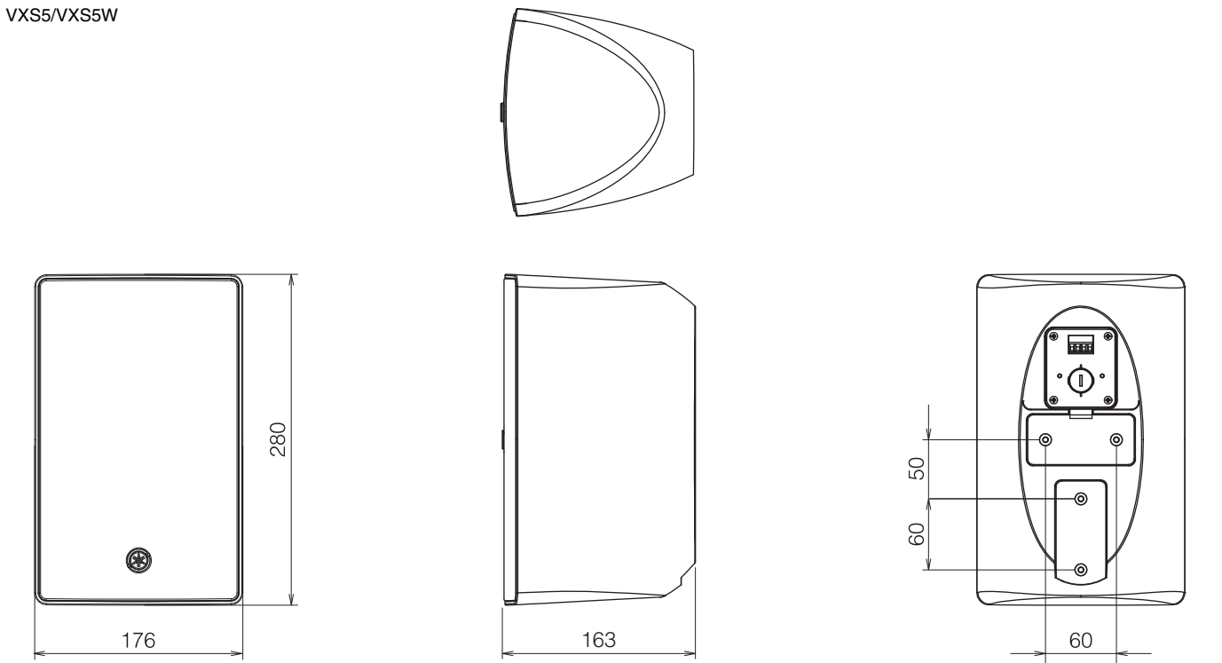
VXS5/VXS5W
