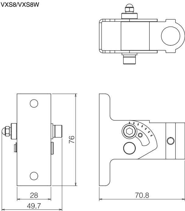
VXS8/VXS8W
