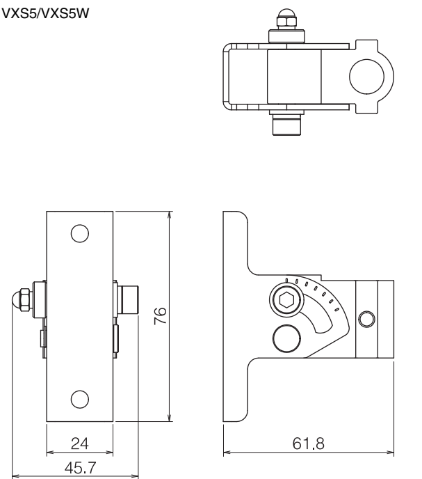
VXS5/VXS5W
