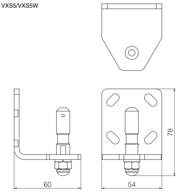
VXS5/VXS5W
