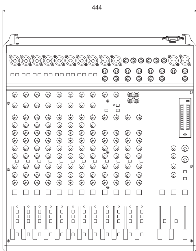
上面図
