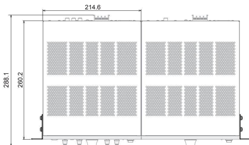
上面図
