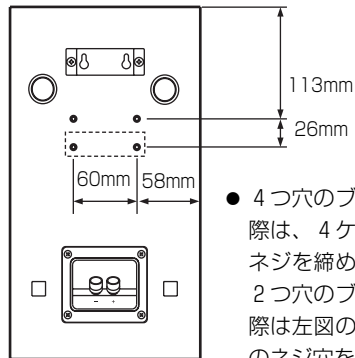
<スピーカー背面図>
