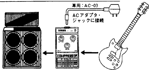
EX. 1 1台のアンプで音を出す一般的な接続例
