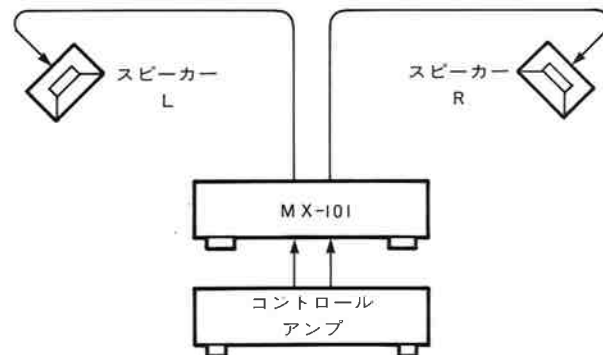
本機を2チャンネル(2 AMP)で使用する場合のシステム例
