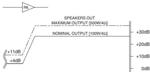
レベルダイアグラムのパワーアンプ出力部分(右端)
