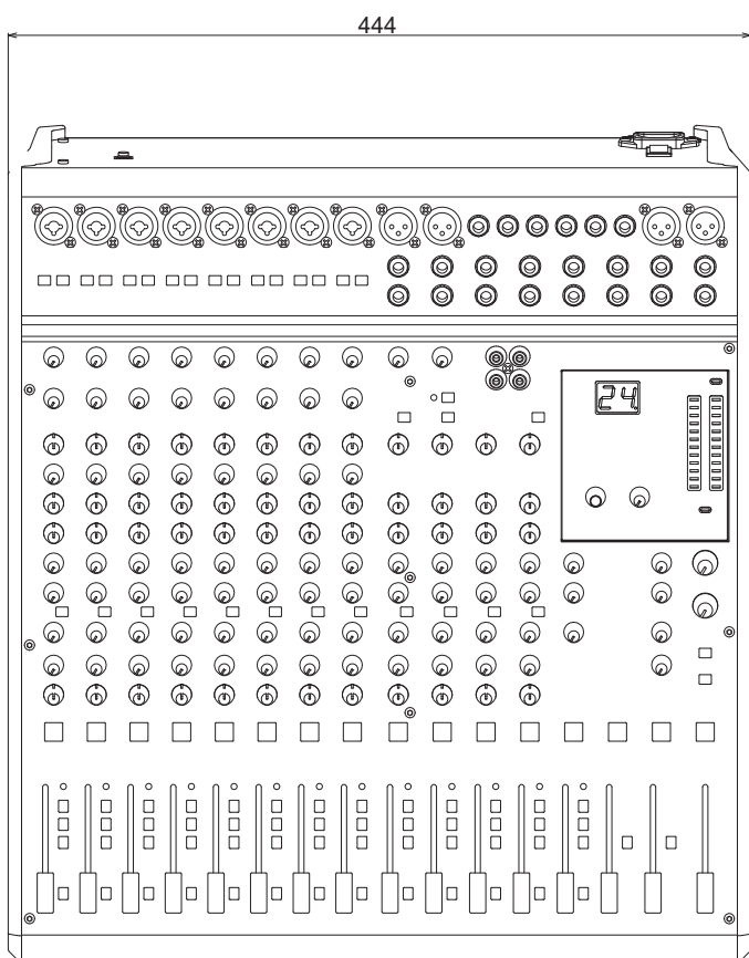
上面図
