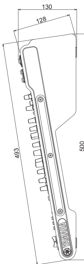
側面図
