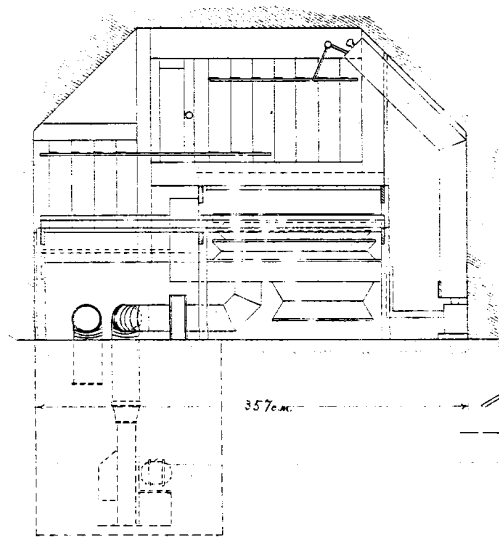
正面圖
